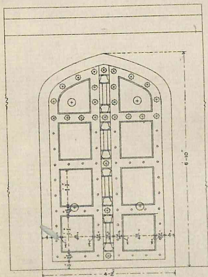
ELEVATION
